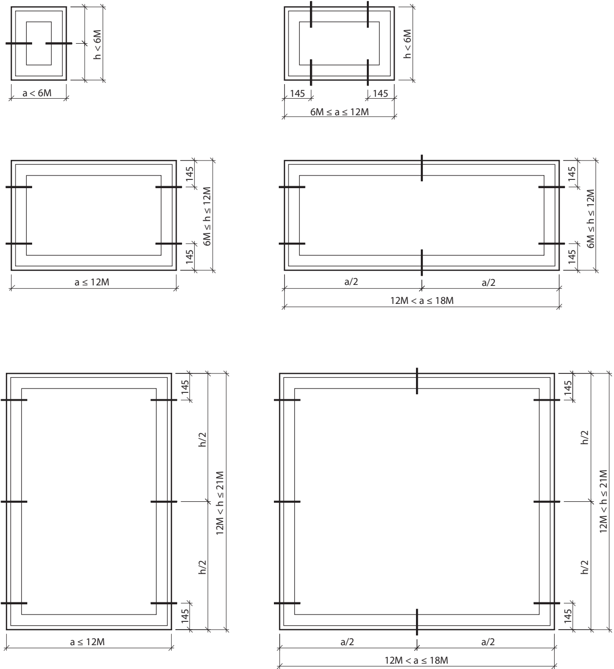
Kuva 36. Sivusaranoidun ja kiinteän puuikkunan ja tuuletusluukun kiinnityskohtien lukumäärä ja sijainti. Kuvat ovat ohjeellisia. Pysty- ja vaaka-kappaleiden keskellä oleva kiinnityskohta voi kuvista poiketen sijaita myös keskitason ala- tai yläpuolella, jos tämä on esimerkiksi heloituksen, jakokarmien tai korvausilmaventtiilien kannalta välttämätöntä.
